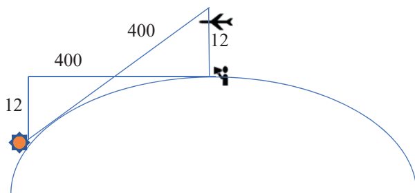
ILUSTRACJA 7 Schemat kierunku obserwacji horyzontu z różnych wysokości.
