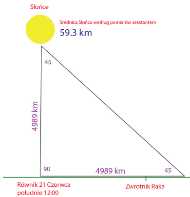
ILUSTRACJA 2 Schemat pomiaru odległości słońca od ziemi wg Volivy.
