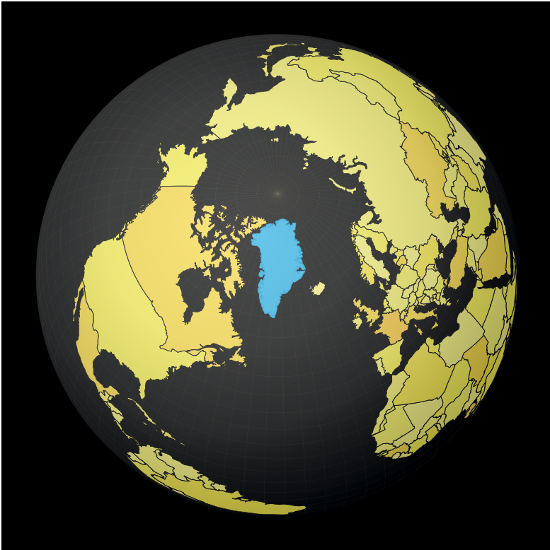
ILUSTRACJA 15A Kula ziemská widziana od strony bieguna północnego.
