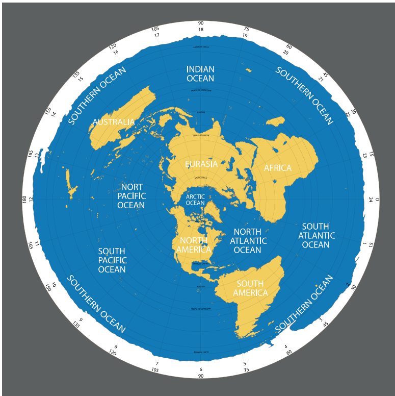
ILUSTRACJA 15C Mapa płaskiej ziemi.
