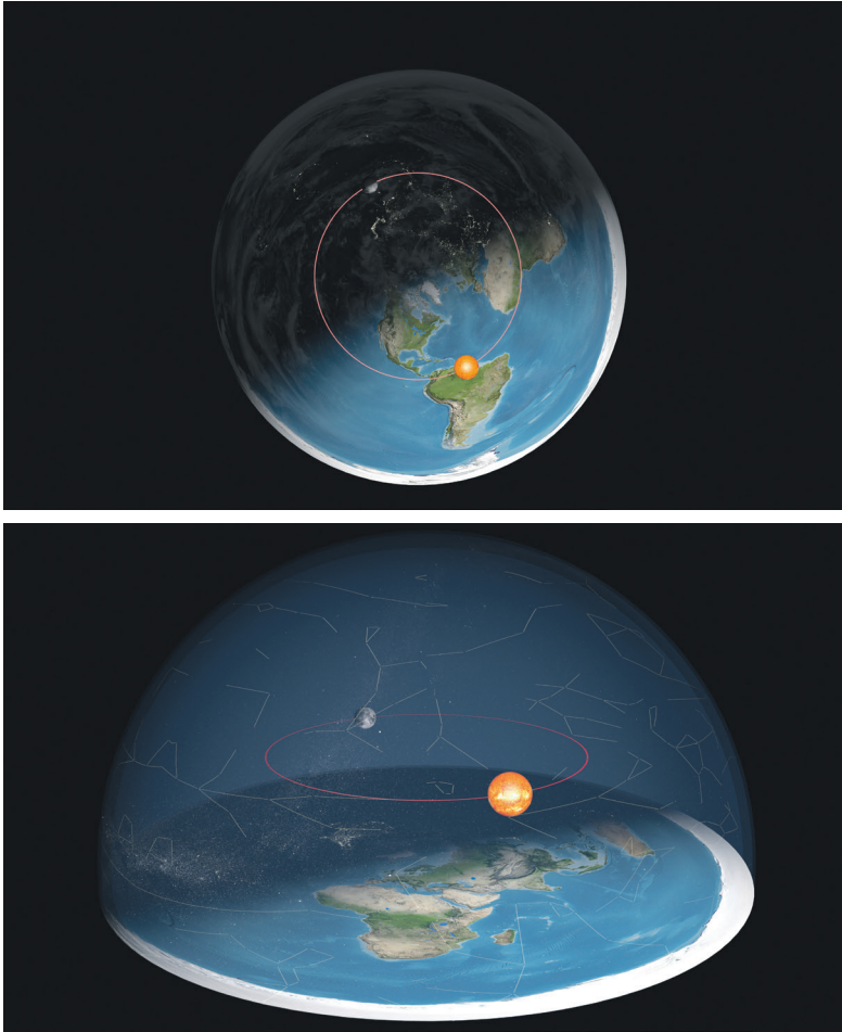
ILUSTRACJA 10 Słońce i księżyc nad płaską ziemią – rzut z góry oraz słońce i księżyc pod firmamentem nad płaską ziemią – spojrzenie z boku.
