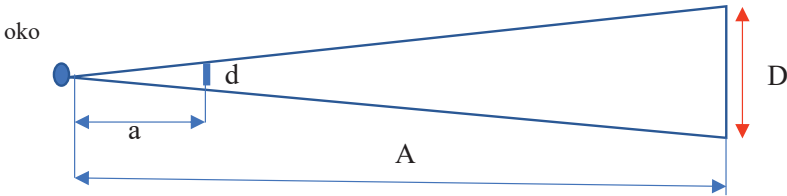
ILUSTRACJA 4 Metodyka wyliczenia średnicy słońca.
