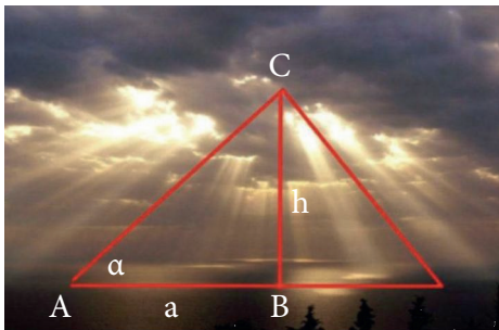
ILUSTRACJA 3 Schemat pomiaru odległości słońca od ziemi wg Volivy.
